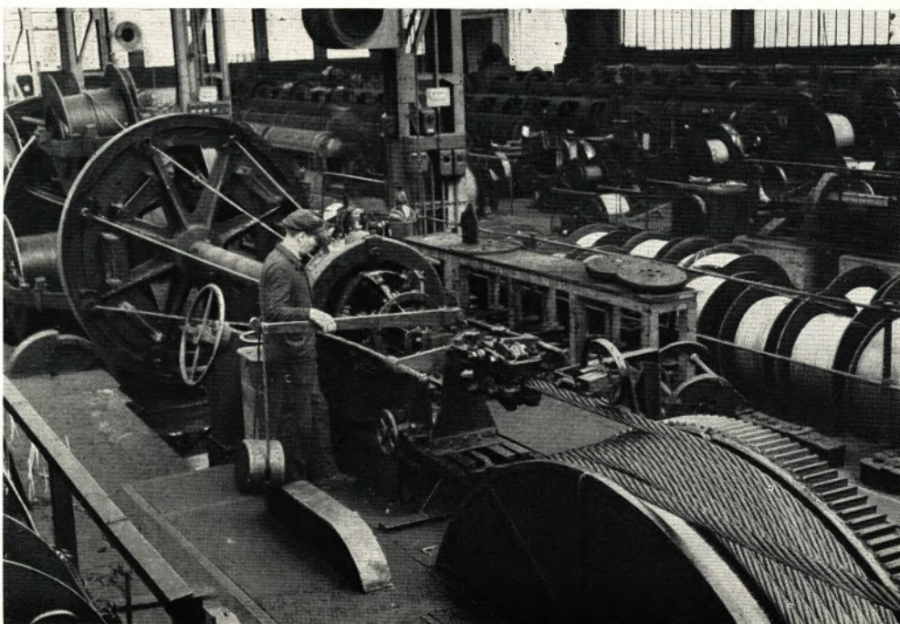
▼ Heute ist die Herstellung von Drahtseilen weitgehendst mechanisiert. Auf verschiedenen Maschinen werden nacheinander Litzen und Seile geschlagen. Bild: Eine Seilschlagmaschine unseres Gelsenkirchener Werkes.
